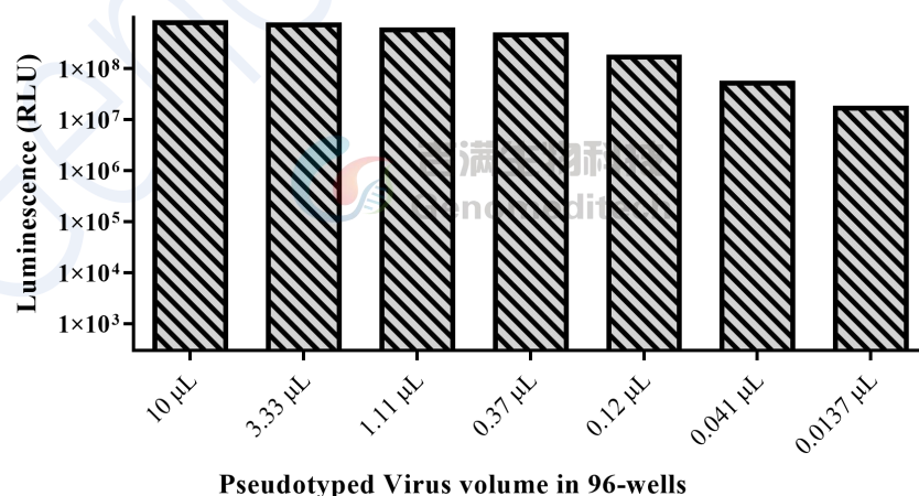
图2 吉满 SARS-CoV-2 Spike S 蛋白(NB.1.8.1)突变型假病毒感染 HEK293T-ACE2 测定 Luciferase 数值
